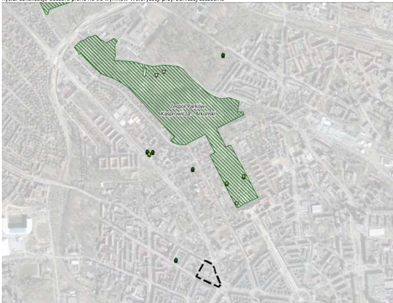
Rys.2. Lokalizacja obszaru planu na tle wyników Waloryzacji przyrodniczej Szczecina
